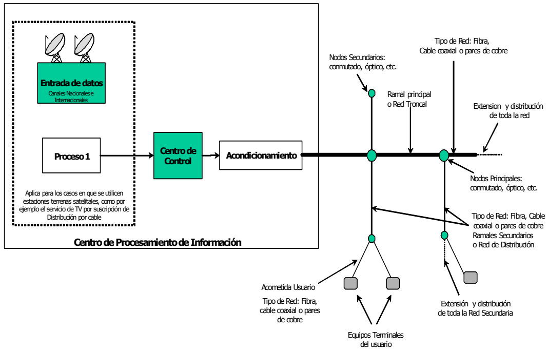
Diagrama de Red Alámbrica
